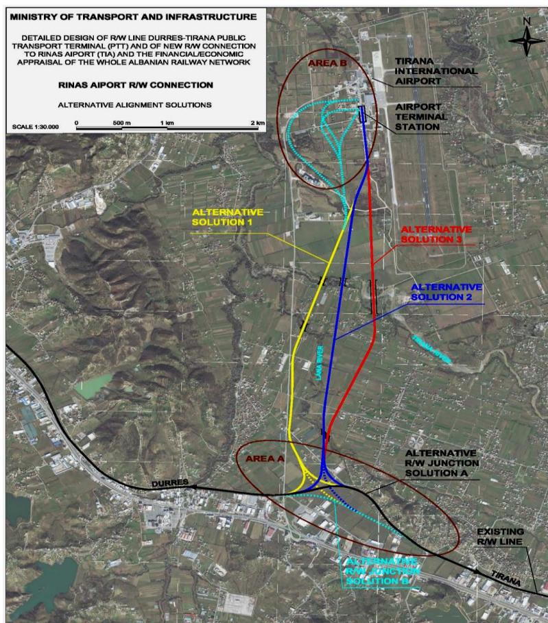
Figura 2. Alternativat për shtrirjen e linjes hekurudhore për në aeroporti e Rinasit Alternativa 2 është zgjidhja e propozuar
